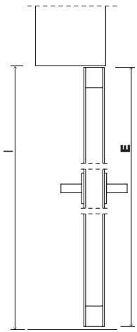
Coupe vertical kit sans tête
