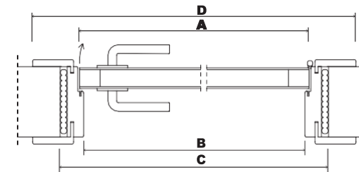
Série Standard Coupe horizontal
