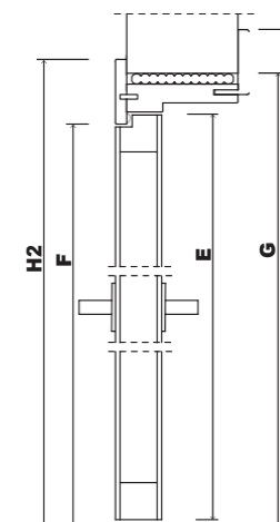
Coupe vertical kit avec tête
