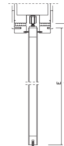
Coupe vertical kit avec tête
